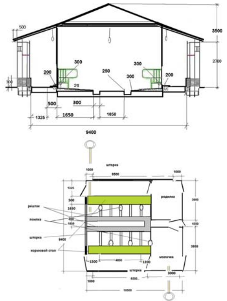
Рис. 6 – Схема молочної ферми на десять корів (с. Українка Апостолівського р-ну)
