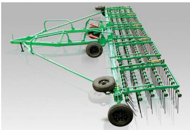
Рис. 1 – Борона пружинна важка БПВ-15 виробництва ТОВ НВП «БІЛОЦЕРКІВМАЗ»
