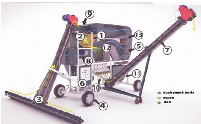
Рис. 3 – Конструкційно-технологічна схема комплексу СОК-25: 1 – зерно; 2 – бункер-накопичувач; 3 – завантажувальний скребковий транспортер; 4 – автомобільні колеса ВАЗ 2108; 5 – циклонно-осаджувальна камера; 6 – пульт управління; 7 – вивантажувальний транспортер; 8 – двигун з імпульсом; 9 – повітропровід; 10 – лотки для сходу фракцій; 11 – бункер відходів; 12 – камера сепарації; 13 – друга осаджувальна камера
