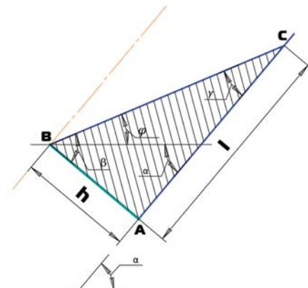
Рис. 1 – Схема переміщення насіння скребком
