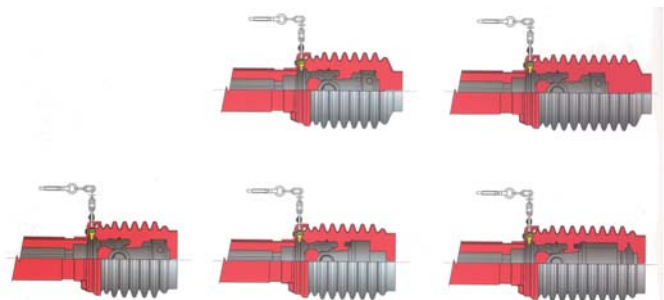
Рис. 3 – Додаткові захисні розтруби Shield Cone Configurations
