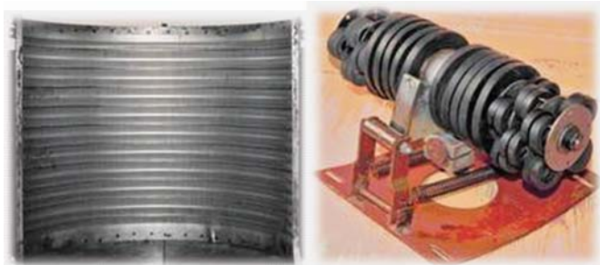
Рис. 2 – Нові конструкції циліндричних решіт, на поперечних, повздовжніх перемичках яких виштампувані рифлі або самі поперечні перемички є виштампуваними рифлями випуклістю всередину решета. Розробники: д-р техн. наук, проф. Тіщенко Л.М., д-р техн. наук, с. н. с. Гончаров Є.С., канд. техн. наук, с. н. с. Прилуцький А.Н., інж. Пуха В.М.
