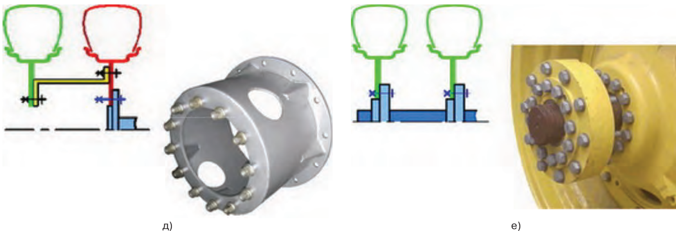
Рис. 5 – Механізми здвоювання: а – м'які «З» зачепи; б – м'які «К» крюки; в – м'які «Р» центральні ригелі; г – жорсткі «М» муфти; д – жорсткі «Б» барабани; е – жорсткі «Д» дві маточини
