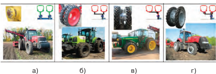
Рис. 4 – Системи здвоювання коліс: а – одинарні; б – зварні; в – напівроз'ємні; г – універсальні
