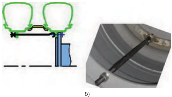
Рис. 3 – Системи здвоювання коліс: а – для суцільного обробітку ґрунту; б – для міжрядного обробітку ґрунту
