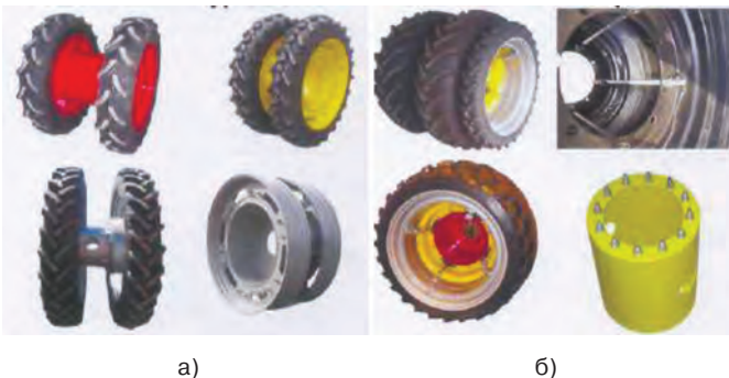
Рис. 3 – Системи здвоювання коліс: а – для суцільного обробітку ґрунту; б – для міжрядного обробітку ґрунту
