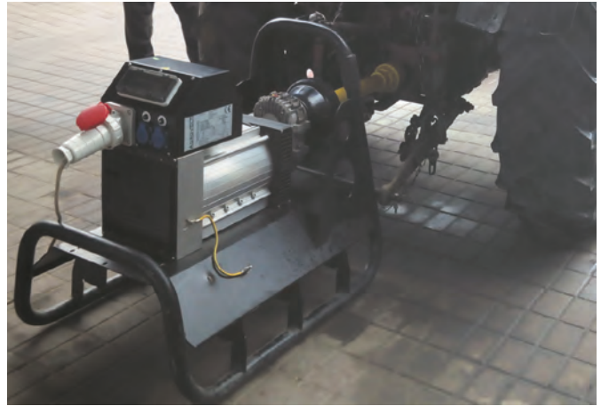
Рис. 2 – Електрогенератор AV38
