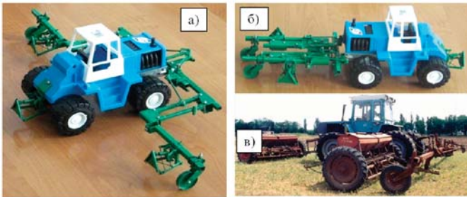
Рис. 2 – Макетний (а і б) та експериментальний (в) зразки тримашинного агрегата на основі напівнавісної зчіпки
