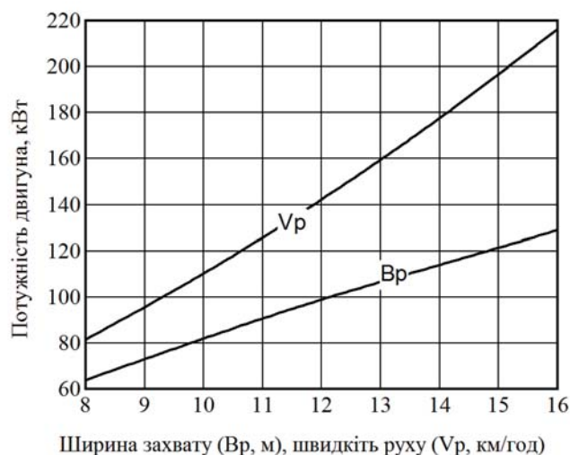
Рис. 1 – Залежність номінальної потужності двигуна трактора від ширини захвату ( B_p ) і робочої швидкості руху ( V_p ) МТА
