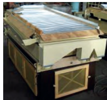
Рис. 7 – Пневмовібростіл для очистки і сортування насіння різних культур ПВСФ-3
