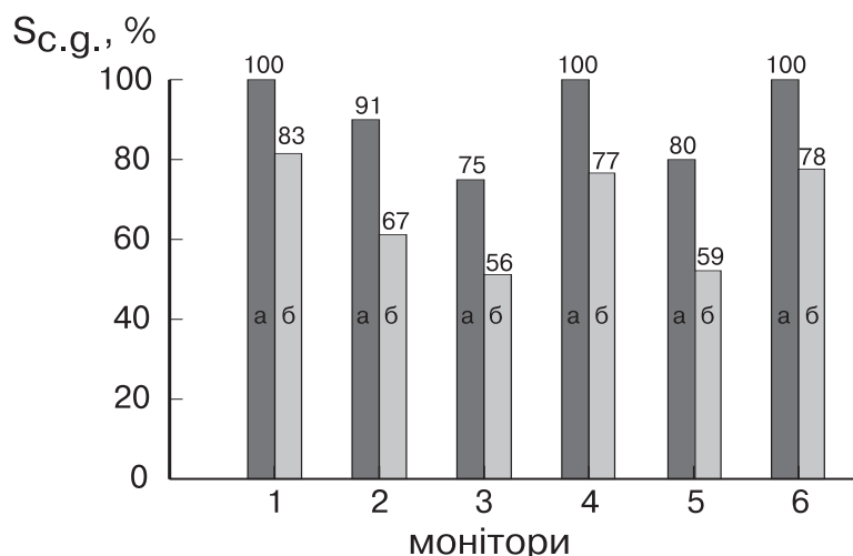
Рис. 3. Колірне охоплення досліджуваних моніторів: 1 — Asus VW202SR (LCD); 2 — Sony Trinitron (CRT); 3 — Samsung R530; 4 — Samsung SyncMaster 2043; 5 — LG Flatron L 194WS; 6 — LG Flatron W1942S; а — колірний профіль «sRGB», б — колірний профіль «Adobe RGB»
