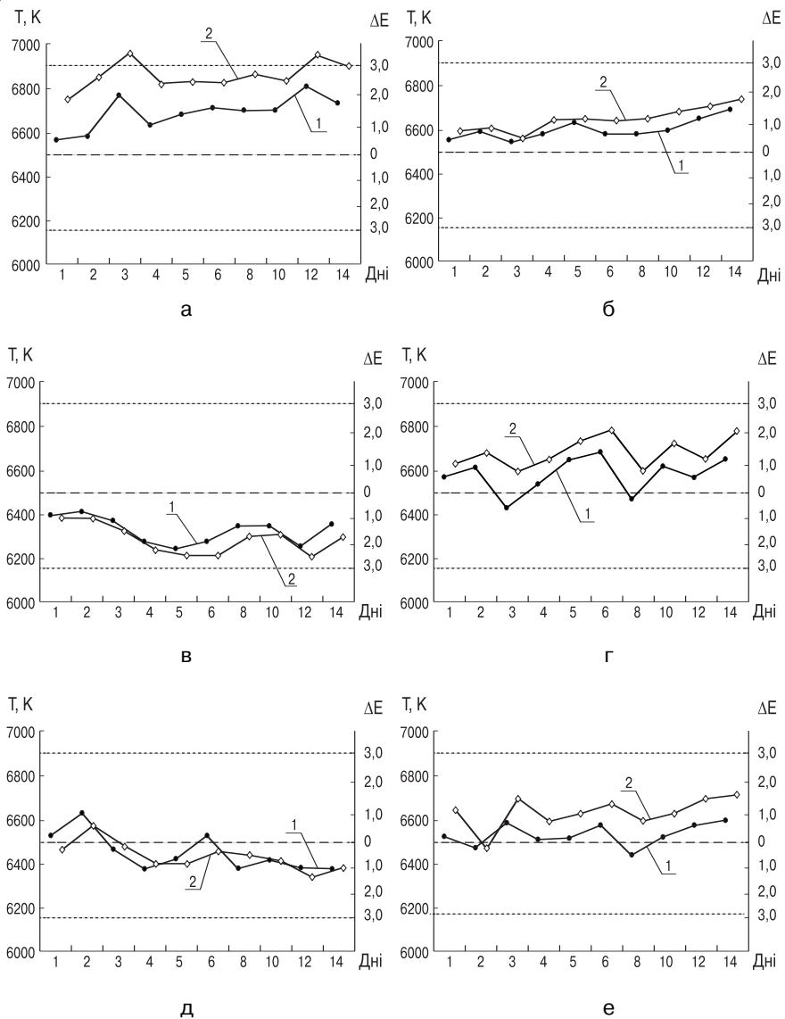
Рис. 4. Розподіл колірної температури за днями: 1 — значення центральної ділянки; 2 — середнє значення дев'яти ділянок; а — Asus W202SR (LCD); б — Sony Trinitron (CRT); в — Samsung R530; г — Samsung SyncMaster 2043; д — LG Flatron L 194WS; е — LG Flatron W1942S
