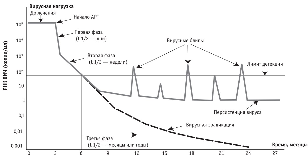
Рис. 1. Схема снижения вирусной нагрузки после начала АРТ [46]
