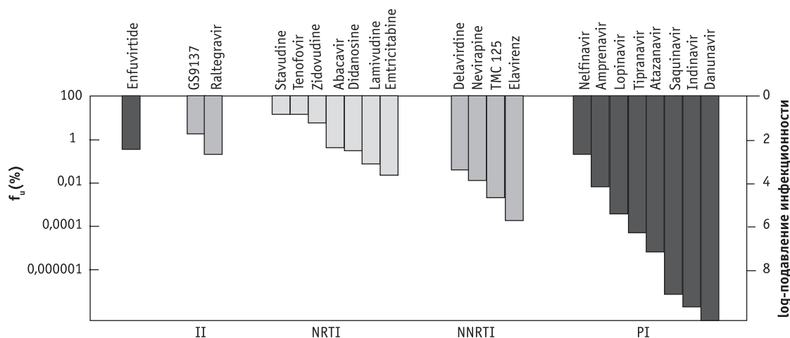
Рис. 2. Относительная эффективность противовирусных препаратов при максимальных концентрациях ( C_{max} ). Относительная эффективность равна логарифму уменьшения инфекционности при клинически значимых концентрациях ( 1/f_u ) [48]
