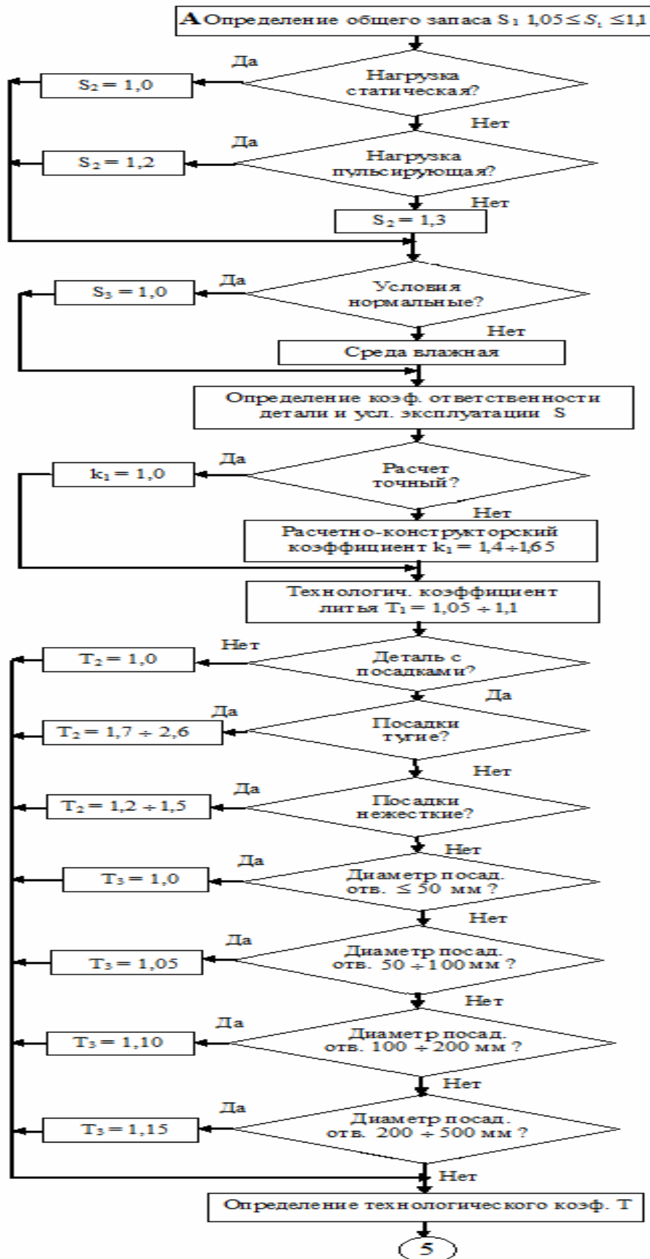
Рис. 3. Алгоритм определения базовых значений показателей качества
