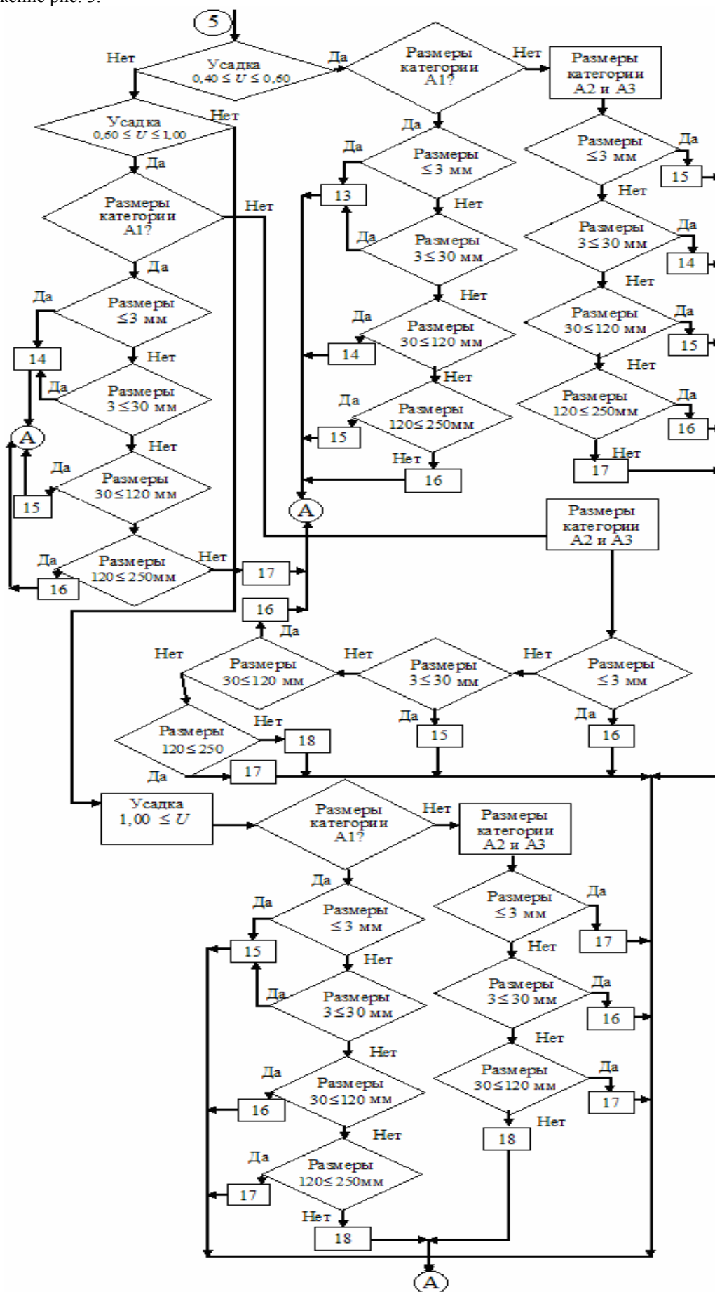
Рис. 3. Алгоритм определения базовых значений показателей качества
