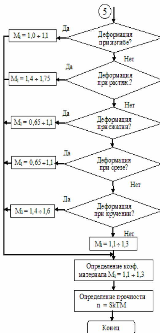
Рис. 3. Алгоритм определения базовых значений показателей качества
