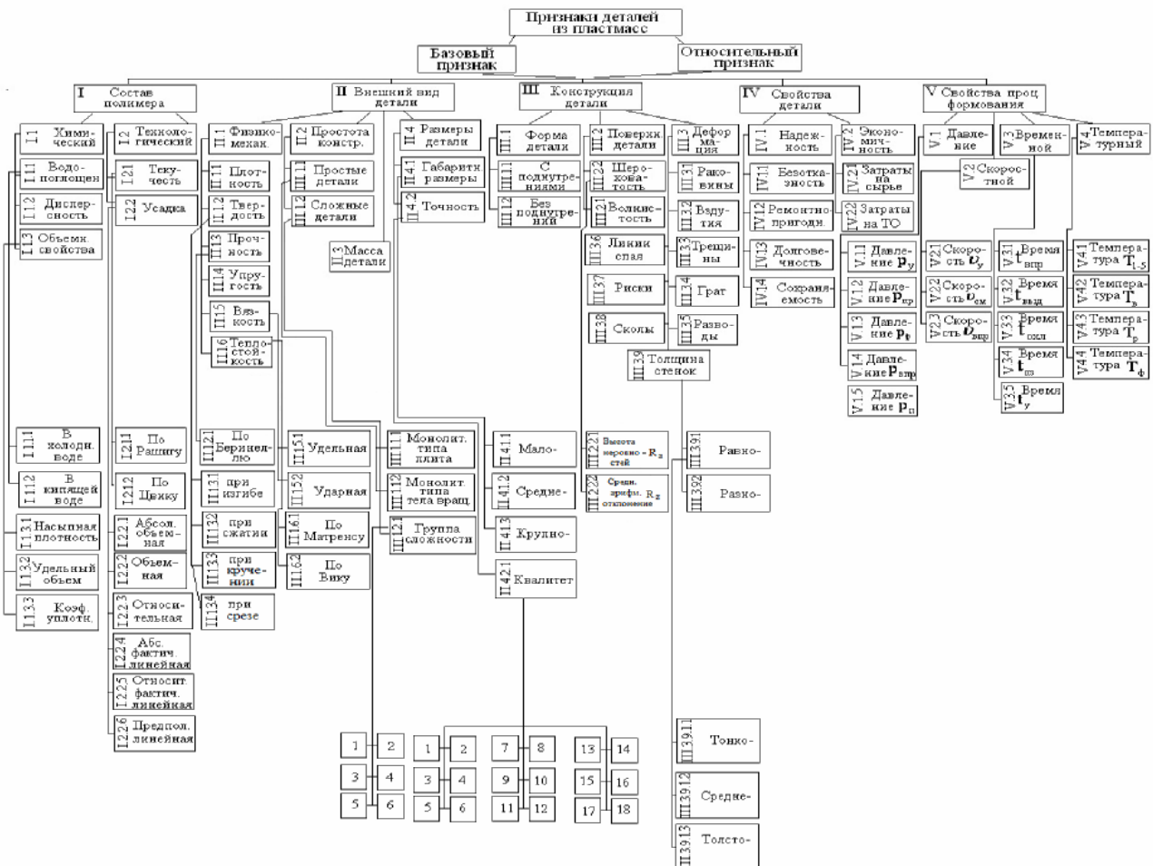
Рис. 1. Граф признаков качества деталей из пластмасс
