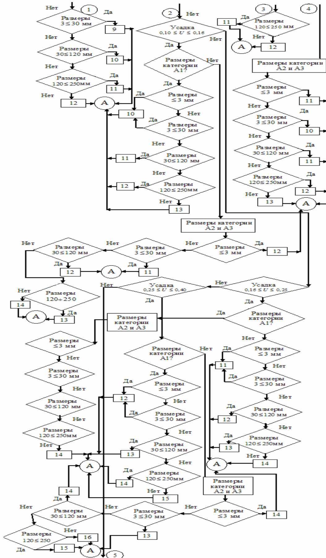
Рис. 3. Алгоритм определения базовых значений показателей качества
