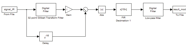
Рис.15. Модель виділення обвідної сигналу
