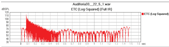
Рис. 4. Результати вимірювання ЕЧЗ для аудиторії з ЧД 22,05 кГц
