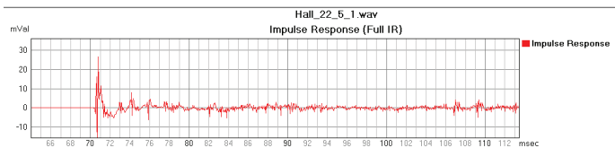
Рис. 7.Результати вимірювання ІВ для коридору з ЧД 22,05 кГц
