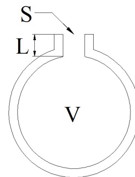
Рис. 5. Резонатор Гельмгольца
