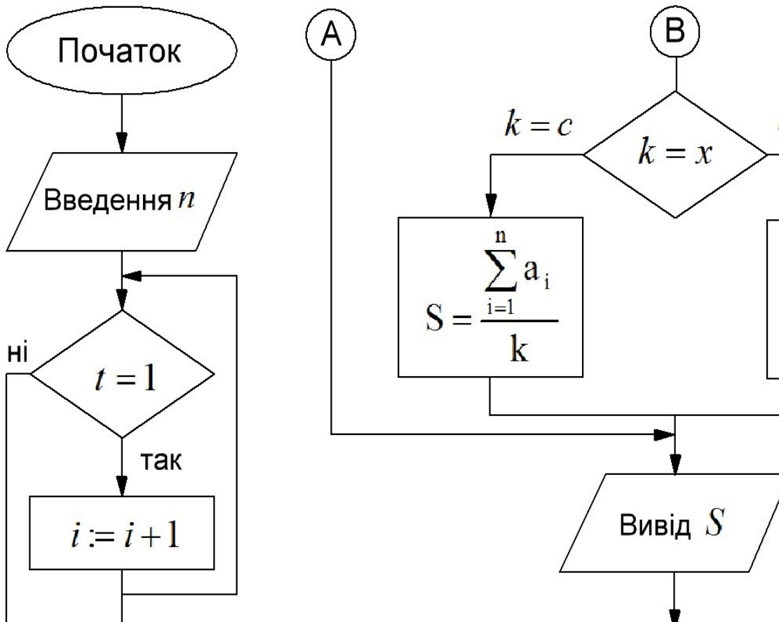
Рис. 3. Алгоритм автоматизованого підрахунку SMD компонентів у стрічках із застосуванням оптопари
