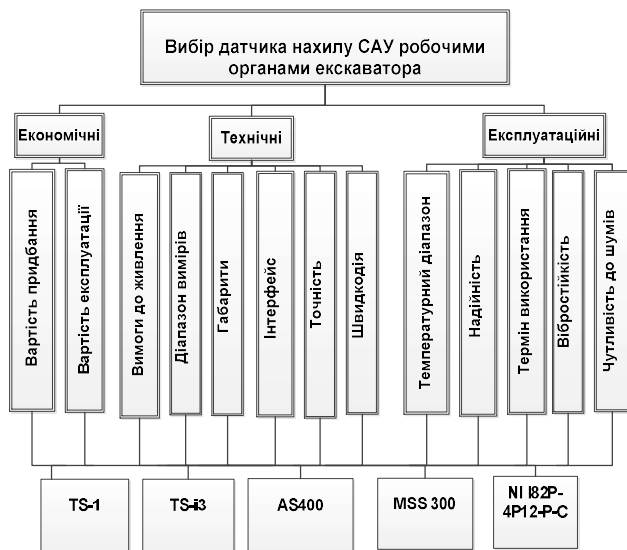
Рис. 1. Структурна модель вибору датчика нахилу системи автоматичного управління робочими органами екскаватора
