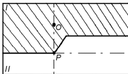
б) із ламаною правою ділянкою світлотіньової межі
