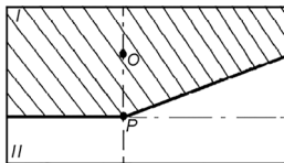
а) із похилою правою ділянкою світлотіньової межі
