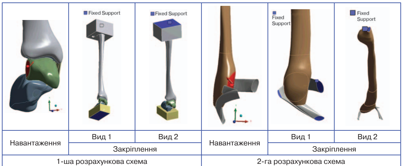
Рисунок 4. Прикладене навантаження та закріплення (спрощені досліджувані геометричні моделі)
