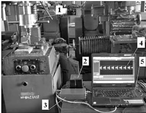
Рис. 7. Вигляд експериментальної установки: 1 – Пристрій для реверсивного свердління ПКМ, 2 – підсилювач, 3 – аналогово-цифровий перетворювач, 4 – вигляд отриманого вібраакустичного сигналу, 5 – ЕОМ
