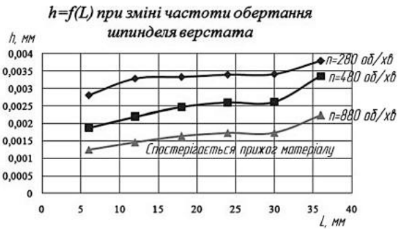
Рис. 10. Графік h = f(L) для ступінчатого свердла
