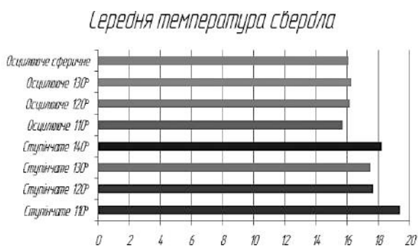
Рис. 17. Діаграма середньої температури інструменту різної конструкції
