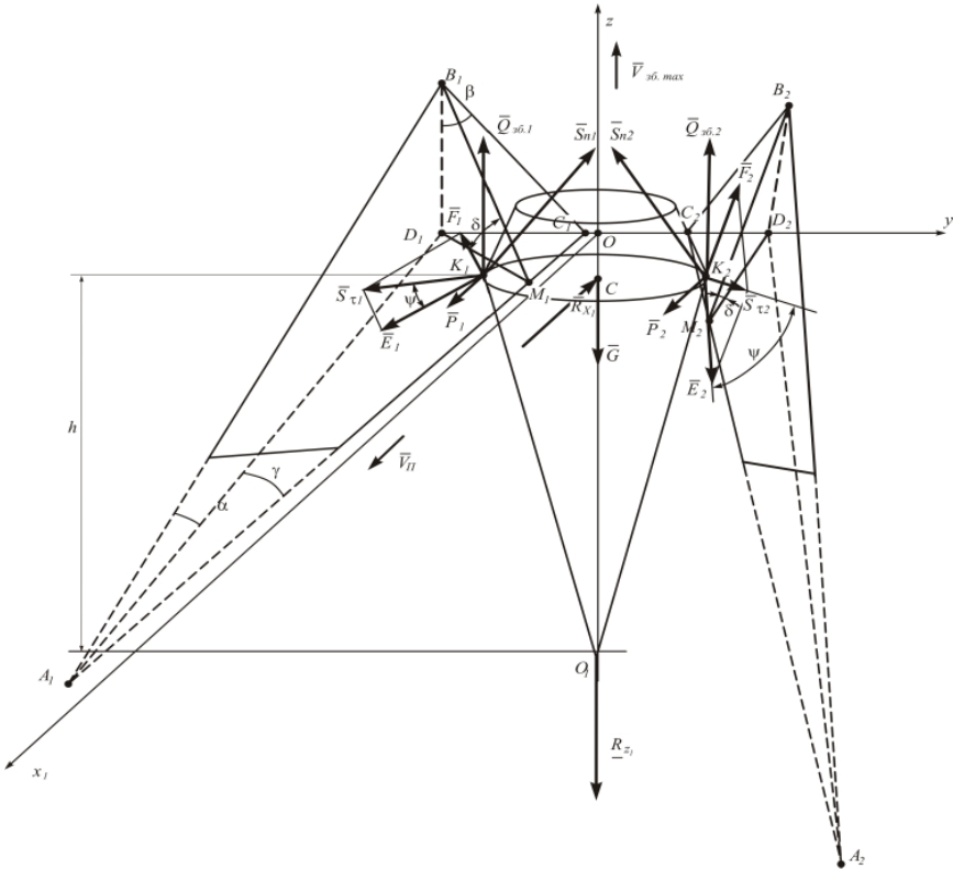
Рисунок 1 – Еквівалентна схема ударної взаємодії вібраційного викопувального робочого органу з коренеплодом, закріпленим у ґрунті
