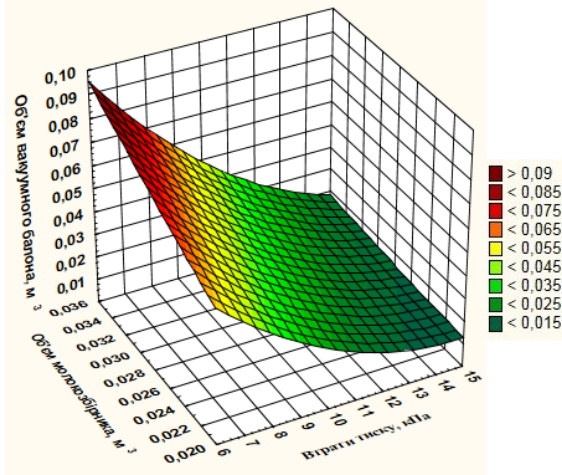
Рисунок 1 – Залежність об'єму вакуумного балона ( V_B ) від об'єму молокозбірника ( V_M ) та втрат вакуумметричного тиску ( \Delta p_B ) за його початкового рівня у вакуумній мережі p_{ПВ}=47 кПа, за умови t \times k_v = \text{const}
