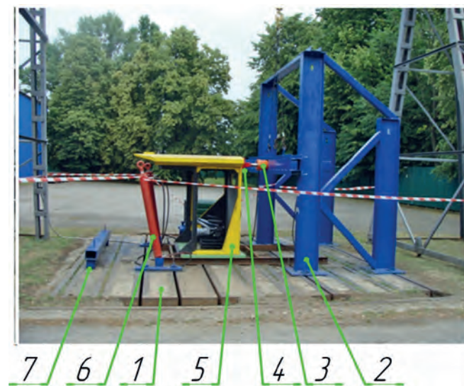
1 - силова підлога; 2 - бічні опори; 3 - гідроциліндр горизонтального навантаження; 4 - брус навантажувальний; 5 - випробовувана кабіна; 6 - гідроциліндри вертикального навантаження; 7 - балка силова вертикального навантаження
