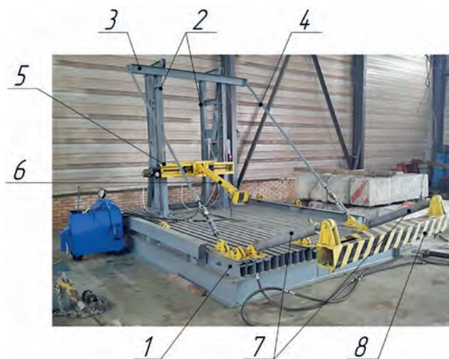
Рисунок 5 – Стенд фірми «Спецавтотехніка» для проведення випробувань кабін статичним горизонтальним та вертикальним навантаженнями [9]
