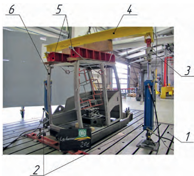
Рисунку 3 – Стенд фірми «Lochmann» для проведення випробувань кабін статичним вертикальним навантаженням [7]
