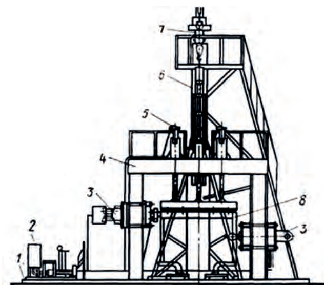
Рисунку 4 – Стенд Челябінського філіалу НАТІ для проведення випробувань кабін динамічним та статичним навантаженням [8]
