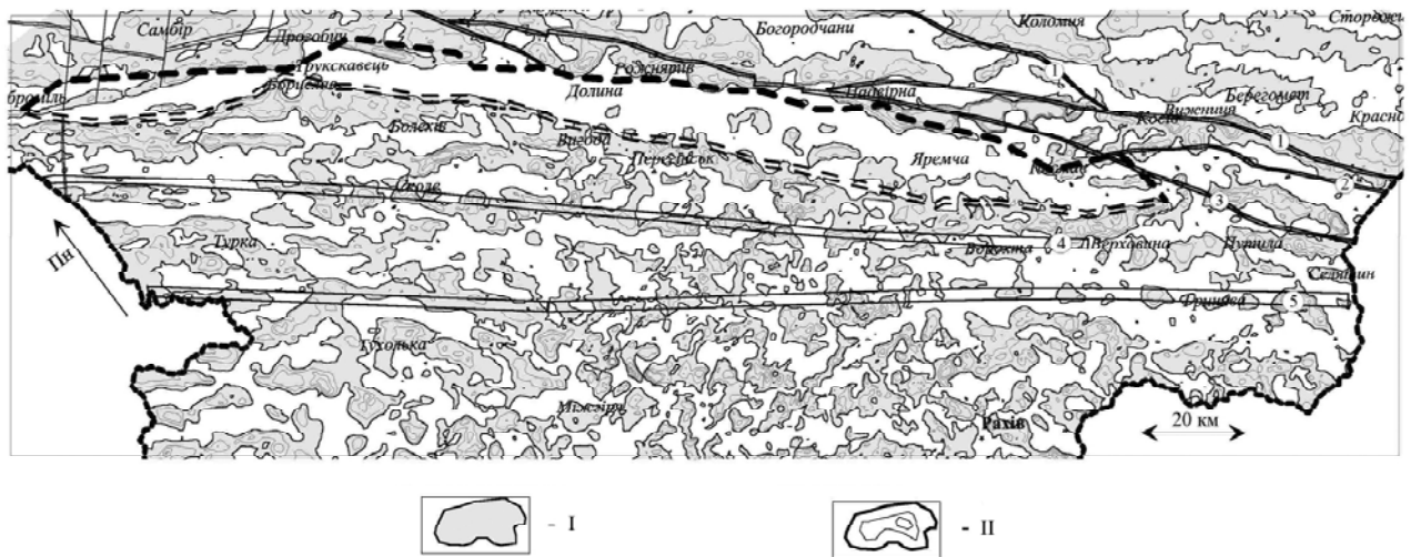
Рис. 4. Додатні локальні аномалії поля сили тяжіння (радіус осереднення – 5000 м): I – додатні аномалії поля сили тяжіння; II – додатні аномалії магнітного поля, переріз ізоліній – 2 нТл. Умовні позначення щодо елементів тектоніки див. на рис. 1
