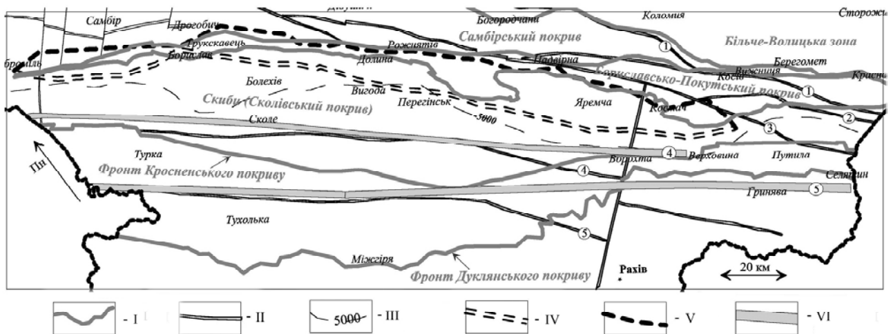
Рис. 1. Елементи тектоніки основи Бориславсько-Покутського покриву і прилеглих зон: I – фронти покривів; II – глибинні розломи 1–5: 1 – Калуський, 2 – Шепітський, 3 – Стрийський, 4 – Сколівський, 5 – Славський; III – глибина підшови Скибового покриву за ізогіпсою – 5000 м (елементи з тектонічної карти під ред. Глушка В.В., Круглова С.С.); IV – Вигодський розлом; V – Передкарпатський розлом (Передкарпатський грабен за картою рельєфу доальпійського підложа Українських Карпат (Біліченко В.Я.)); VI – трасування розломів за гравіметричними матеріалами: 4 – Сколівський, 5 – Славський
