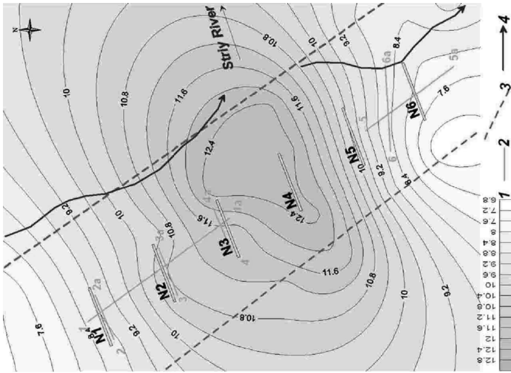
Рис. 3. Карта мощности рыхлых отложений на участке строительства мостового перехода через р. Стрый. 1 – шкала мощности рыхлых отложений (метры); 2 – профили георадарного зондирования N1–6; 3 – тектонические нарушения; 4 – направление миграции подземных вод
