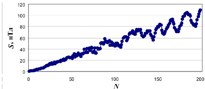
Рис. 2. Залежність точності знімання від параметра розрідження мережі реєстрації N
