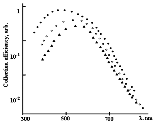
Рис. 5. Зависимость коэффициента собирания от длины волны падающего света для солнечных элементов: \blacktriangle – солнечный элемент типа барьера Шоттки; \circ – солнечный элемент типа n-i-p -переходов; \bullet – солнечный элемент типа двойных n-i-p -гетеропереходов
