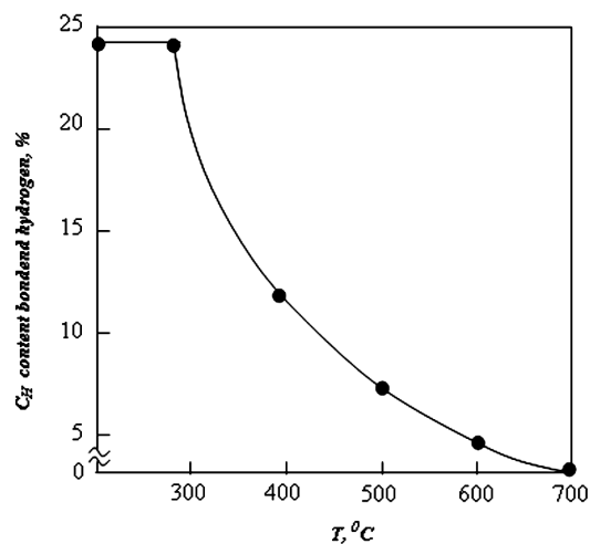
Рис. 3. Зависимость концентрации водорода от температуры отжига T_a
