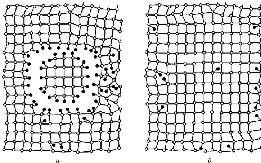
Рис. 2. Схематическая модель для структуры плёнок нк -Si: a – состояние после осаждения; б – состояние после отжига во время t = 1 час и T_a \geq 600 °C
