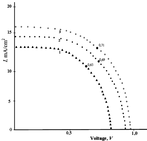
Рис. 4. Характеристики солнечного элемента при освещении 100 \text{ мВт/см}^2 . Кривая 1 для типа барьер Шоттки, кривая 2 для типа n-i-p -гетеропереходы, кривая 3 для типа двойных гетеропереходов
