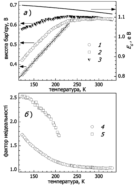
Рис. 3. Температурні залежності висоти бар'єра (а) та фактора неідеальності (б) Mo/n-Si діодів Шотки: 1 – \Phi_{b1} , 2 – \Phi_{b2} , 3 – \Phi_{\text{bef}} , 4 – n_1 , 5 – n_2 . Пунктир – лінійна апроксимація кривої 2. Також наведено температурну залежність ширини забороненої зони Si (а, суцільна лінія)
