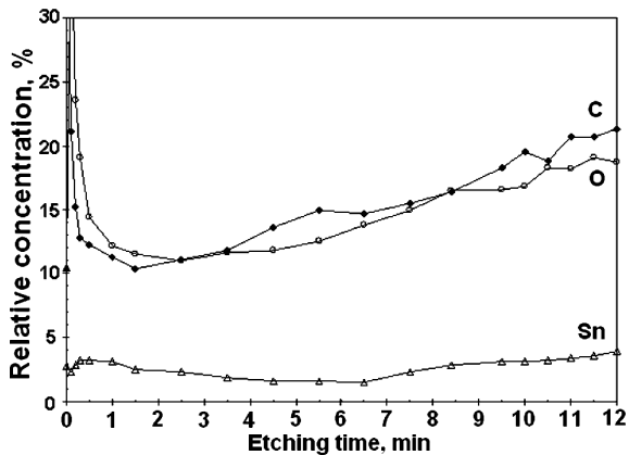
Рис. 4. Розподіл концентрації складових сплаву по товщині плівки від часу іонного травлення
