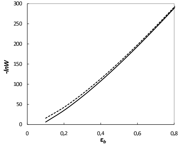
Рис. 4. Логаритм ймовірності іонізації за формулою (17) (суцільна лінія) порівняно з келдишевською формулою (12) без релятивістської поправки (пунктирна лінія), \eta = 1,47 . Урахування кулонівської взаємодії збільшує ймовірність іонізації
