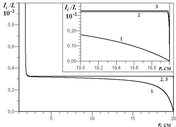
Рис. 6. Частина йонного струму I_i/I в залежності від радіуса в ЖР: 1 – без урахування АП, 2 і 3 – з урахуванням АП при напруженості поля на аноді E_A^* і E_{Af} , відповідно. Розрядний струм I = 100 мА, тиск p = 150 Па
