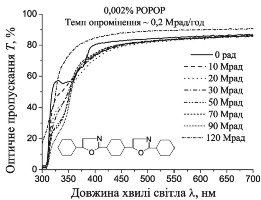
Рис. 2. Оптичне пропускання T зразків із введеними у концентрації 0,002% молекулами РОРОР (1,4-бис-(2-(5-фениллоксазоліл)) – бензолу) у Sylgard-184 в залежності від довжини хвилі світла \lambda для різних доз опромінення D
