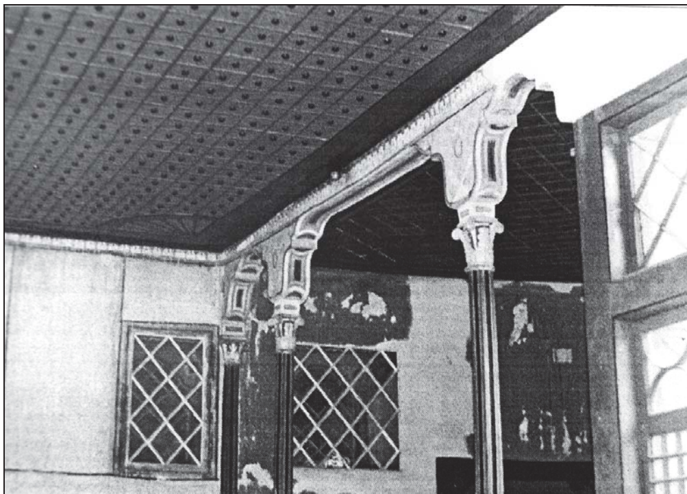
Рис. 1. Общий вид конструкций перекрытия Посольского зала
