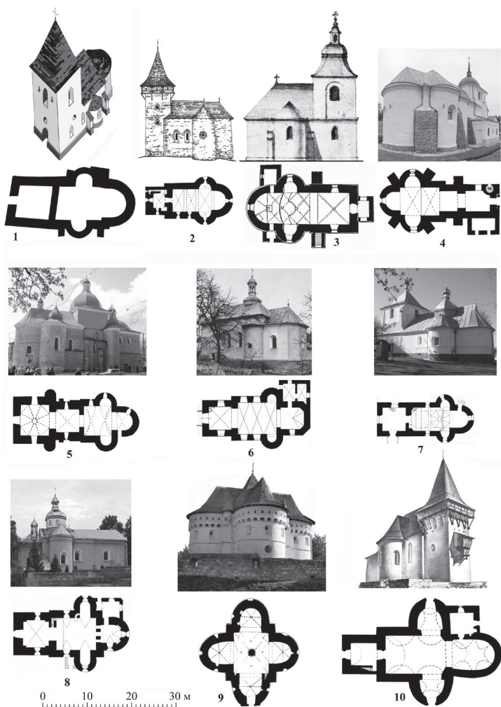
Іл. 2. Оборонні триконхові й тетраконхові православні храми Західного Поділля: 1 — Троїцька церква у м. Кам'яниці-Подільському (реконструкція О. Пламеницької); 2 — Церква в урочищі Монастирок під Бучачем Тернопільської обл. (реконструкція О. Пламеницької); 3 — Іоано-Предтеченська церква у м. Кам'яниці-Подільському (вигляд за креслеником XVIII ст.); 4 — Петропавлівська церква у м. Кам'яниці-Подільському; 5 — Троїцька церква у м. Бережани Тернопільської обл.; 6 — Миколаївська церква у м. Бучач Тернопільської обл.; 7 — Покровська церква в с. Адамівка Хмельницької обл.; 8 — Онуфрійська церква у смт Гусятин Тернопільської обл.; 9 — Покровська церква-замок у с. Сутківці Хмельницької обл.; 10 — Покровська церква-замок у с. Шарівка Хмельницької обл. (реконструкція Є. Пламеницької)
