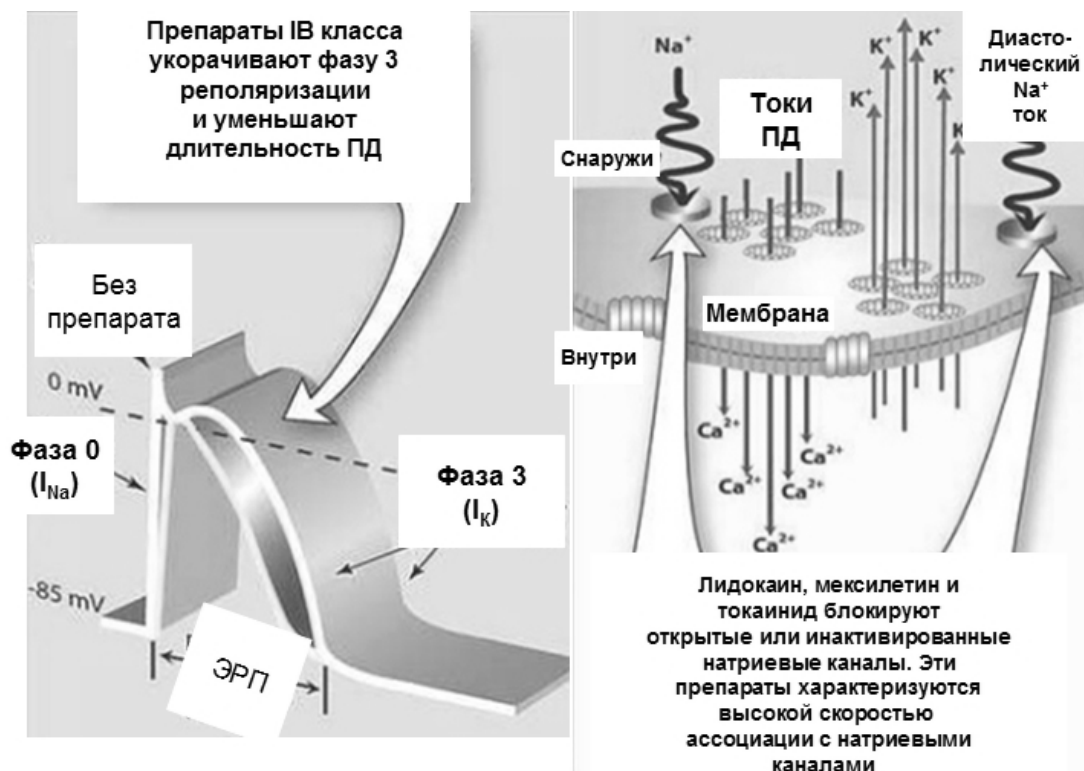
Рис. 3. Механизм действия антиаритмиков класса IB [22].
