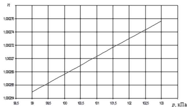
Рис. 4. График зависимости коэффициента преломления воздуха от атмосферного давления для опорных значений температуры t = 20 °С и относительной влажности \phi = 60 %
