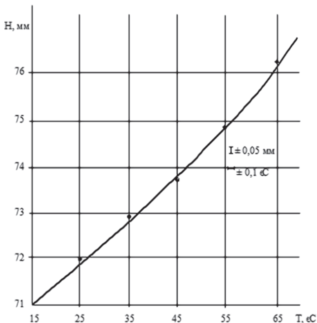
Рис. 3. График зависимости расстояния от оптического отражателя на поплавке до поверхности воды от температуры воды
