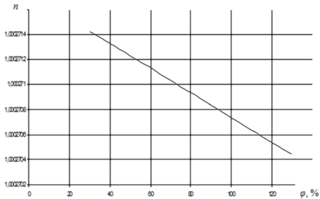
Рис. 6. График зависимости коэффициента преломления воздуха от влажности для опорных значений температуры t = 20 °С и атмосферного давления p' = 101,4 кПа
