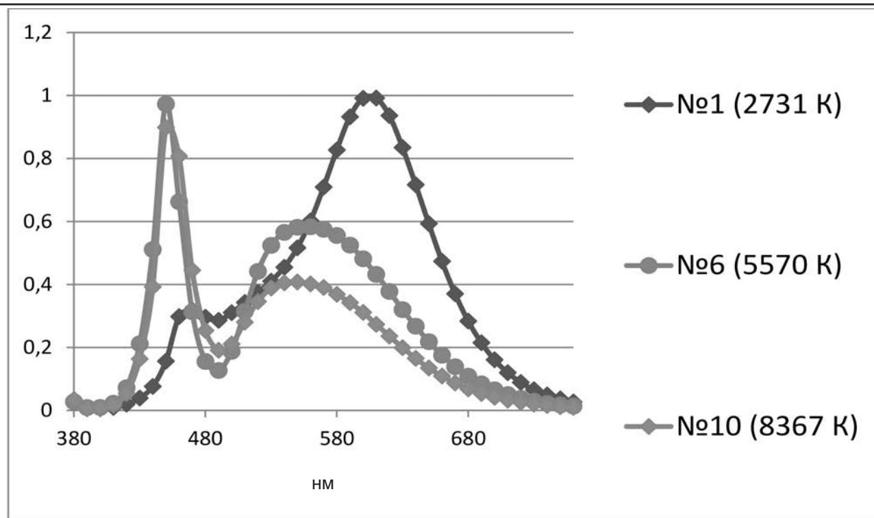
Рис. 1. Нормовані спектри випромінювання світлодіодів із трьома різними T_c : № 1 – 2731 К; № 6 – 5570 К; № 10 – 8367 К
