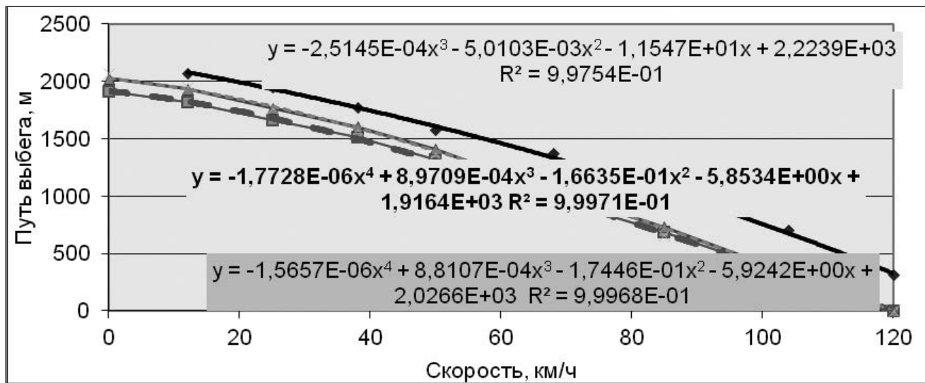
Рис. 3. Полная диаграмма выбега Priora по данным "Авторевю" (сплошная линия) и две диаграммы выбега, рассчитанные предлагаемым методом: по данным "Авторевю" (штриховая) и по данным "За рулем" (треугольные маркеры)
