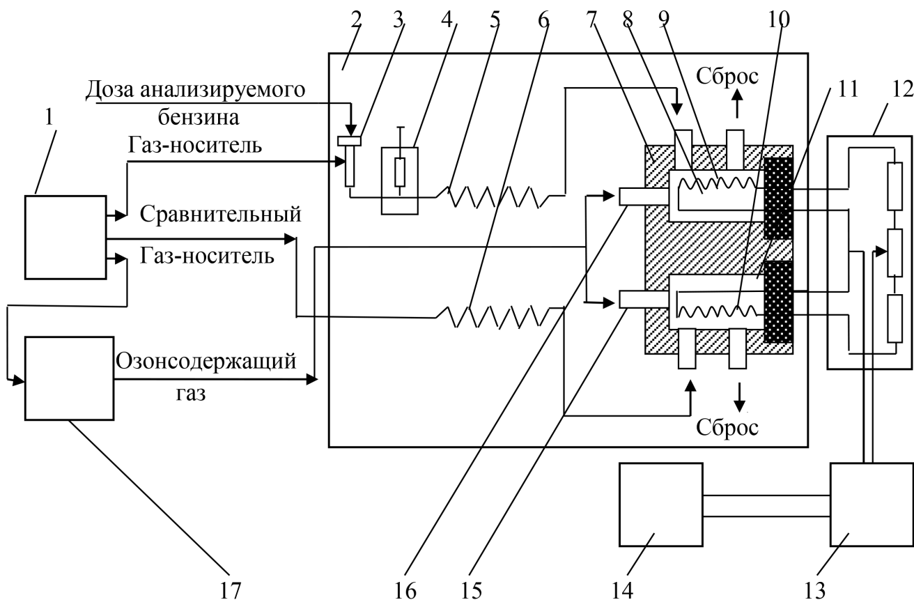
Рис. 1. Установка для определения детонационной стойкости бензинов: 1 – блок подготовки газов; 2 – термостат; 3 – испаритель; 4 – делитель потока; 5 и 6 – полые колонки; 7 – термокондуктометрический детектор; 8 – измерительная камера; 9 и 10 – терморезисторы; 11 – сравнительная камера; 12 – неравновесный мост; 13 – блок управления; 14 – самописец; 15 и 16 – штуцеры; 17 – синтезатор озона
