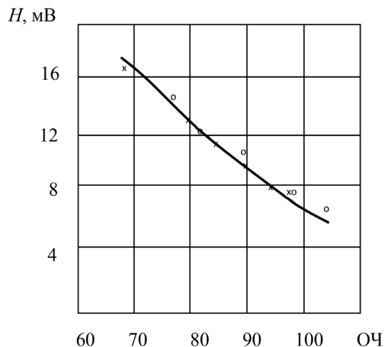
Рис. 2. Градуировочный график: о – контрольное топливо; х – топливо, аттестованное исследовательским методом
