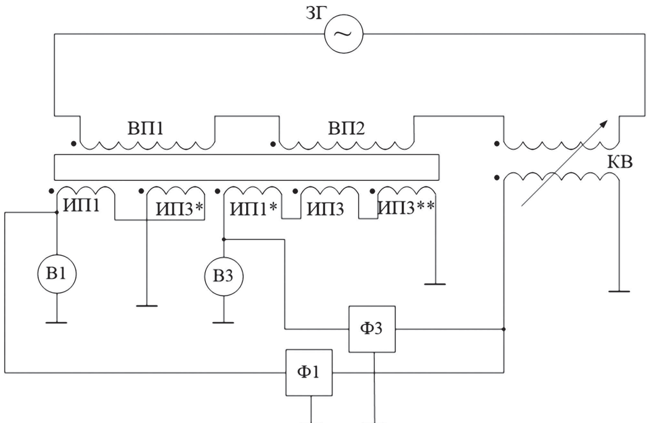
Рис. 3. Схема включения обмоток для выделения 1-й и 3-й гармоник: В1, В3 — вольтметры; Ф1, Ф3 — фазометры; 3Г — задающий генератор; КВ — катушка взаимной индуктивности
