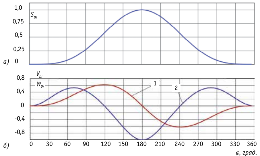
Рис. 3. Графіки залежностей відносних кінематичних параметрів вертикальних повзунів натискної плити від кута повороту кривошипа: переміщення (а); 1 – швидкості, 2 – прискорення (б)
