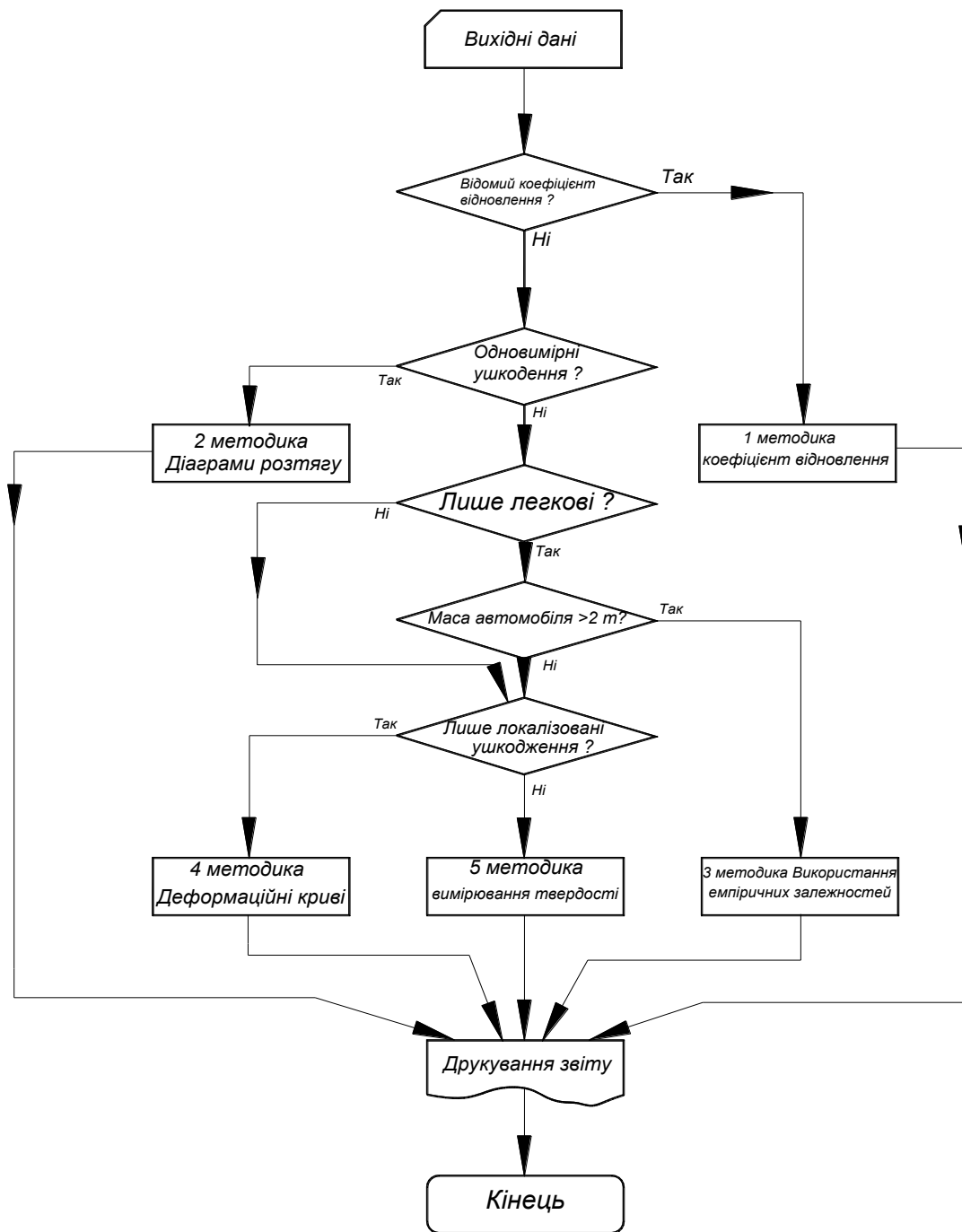
Рисунок 1 – Алгоритм вибору методики визначення швидкостей руху автомобілів
