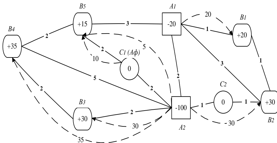
Рисунок 1 – Графічне представлення ТЗ у вигляді дорожньо-транспортній мережі
