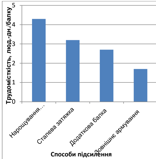
Рисунок 7 – Гістограма трудомісткості підсилення балки варіантами способів
