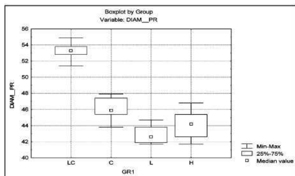
Рис. 2. Діаметральна прочність ФКМ
