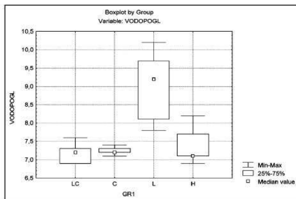
Рис. 3. Водопоглощение ФКМ
