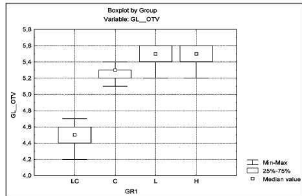
Рис. 1. Глубина отверждения ФКМ
