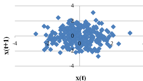
Рис. 3. Псевдофазовий простір ряду випадкових значень
