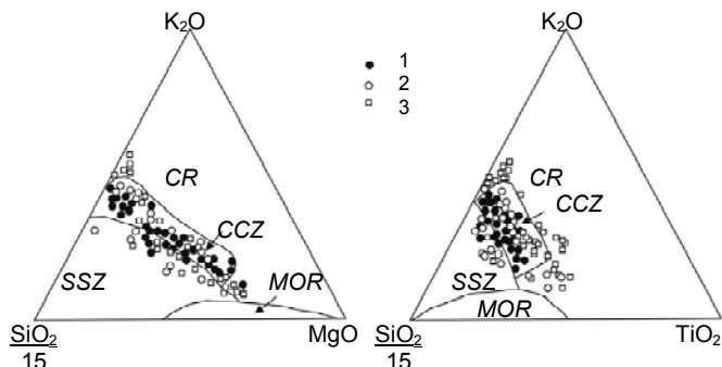
Рис. 3. Базальты Кавказского сектора Альпийского складчатого пояса на диаграмме А. Миясиро [1974] Данные авторов, а также из работ [10], [14]: 1 – Большой Кавказ; 2 – Малый Кавказ; 3 – Восточная Анатолия
