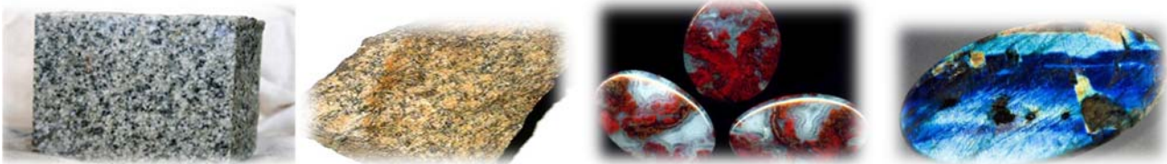
Рис. 2. Белоубинско-Южно-Алтайская зона: граниты, яшма, лабрадорит
