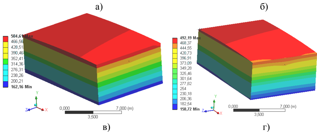
Рис. 2. Розподіл швидкості зміщення частинок ґрунту по осі Z:
