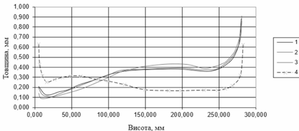
Рис. 3 – Розподіл товщини стінки по висоті пляшки
